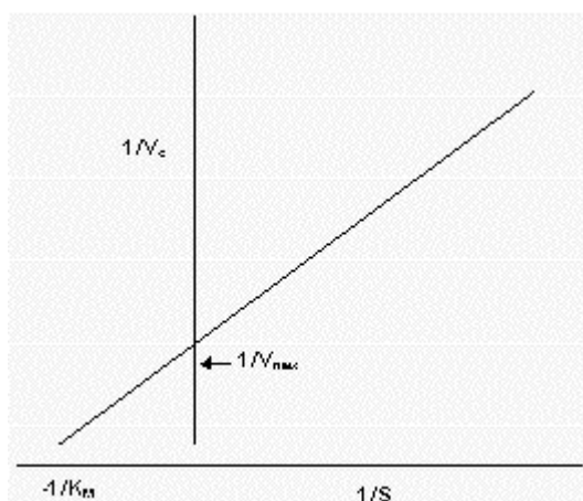
Fig. 3.8. Lineweaver-Burk plot.
