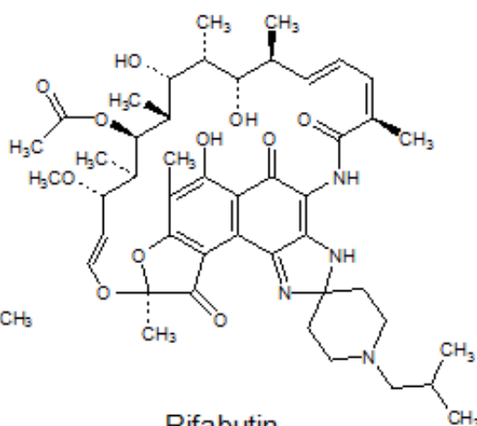
Rifabutin
