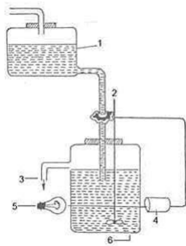
Fig: Turbidostat
