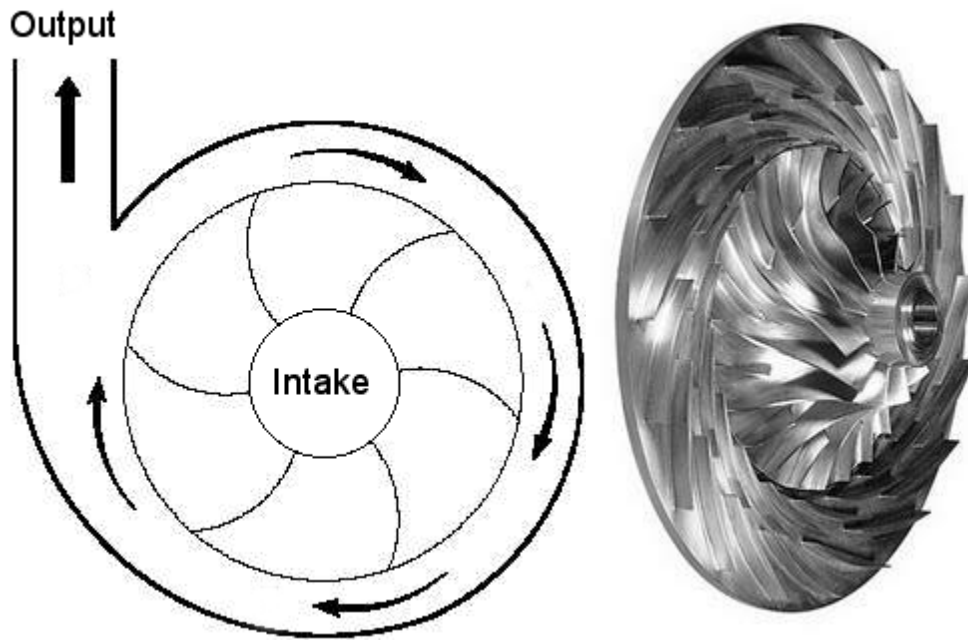
Impeller
