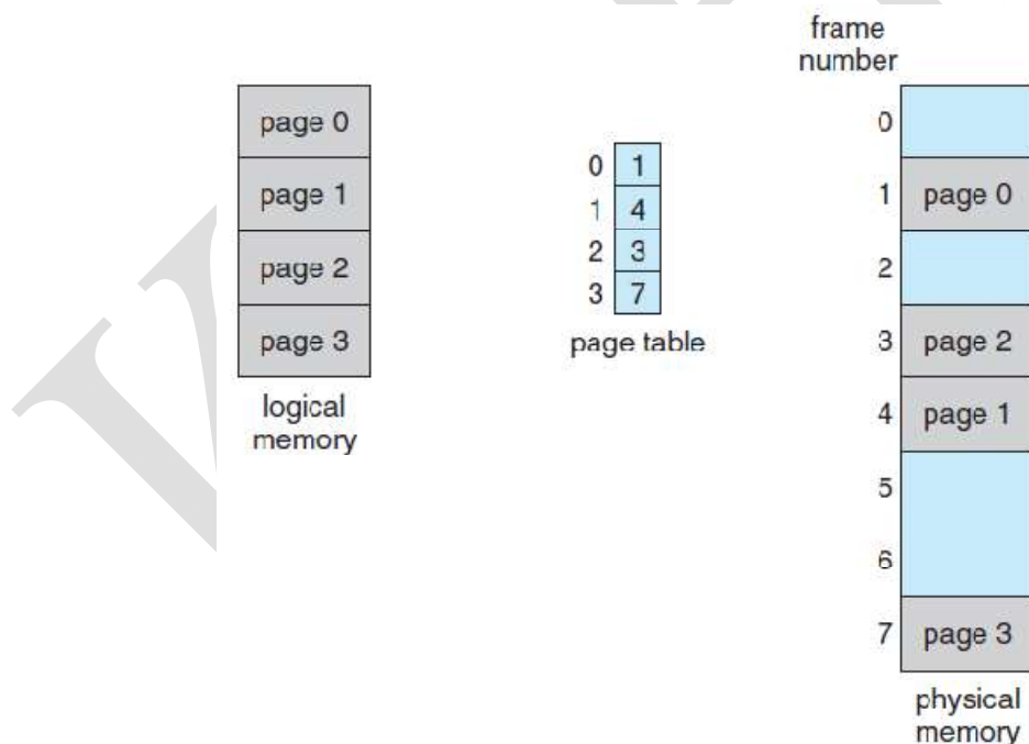
Fig 3.12. Page Table
