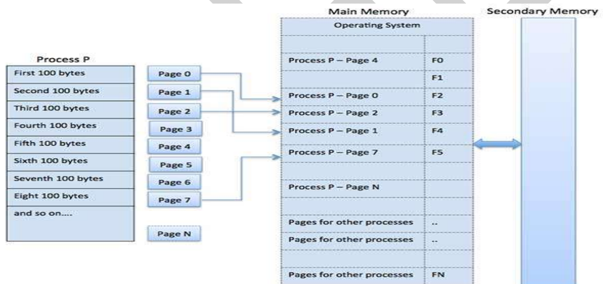
Paging Process
